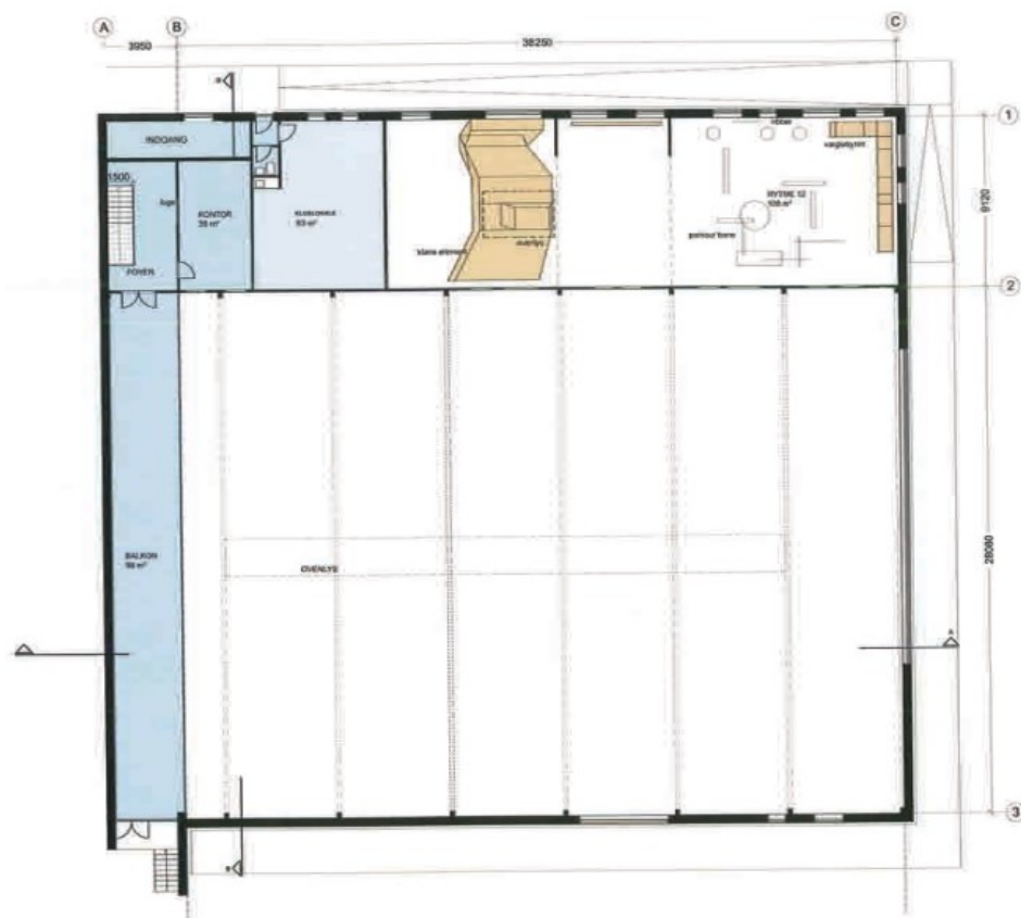
PRINCIP PLAN ØVRE 1:200
