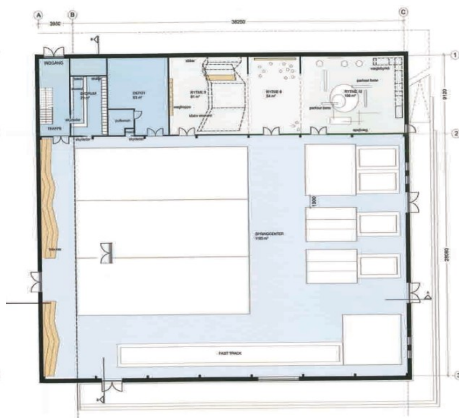
PRINCIP PLAN NEDRE 1:200
